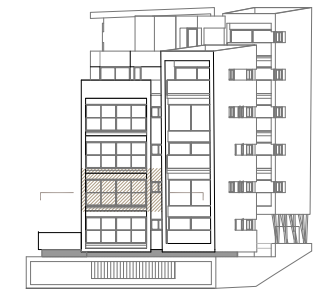
ALZADO RÍA O BURGO
