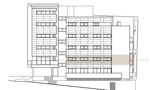
ALZADO LATERAL 02
