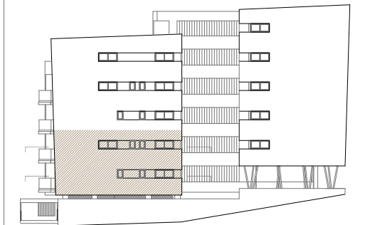
ALZADO LATERAL 01
